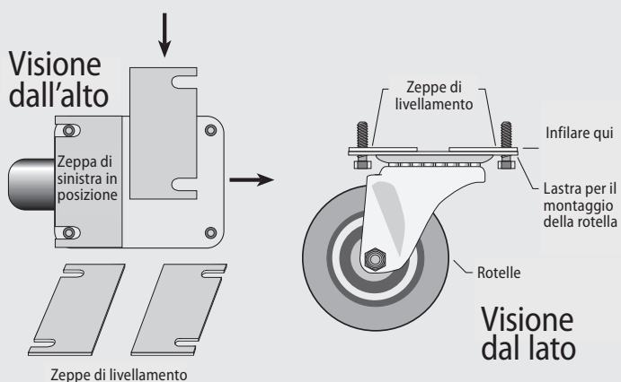
Fig. 3. Rotelle di piattaforma e zeppe. Installare le zeppe a coppie.
