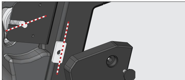
Afb. 3. Lijn de platte randen (aangegeven met de stippellijnen) van de demper en de einddop van de klephouder uit tijdens het opnieuw monteren.
