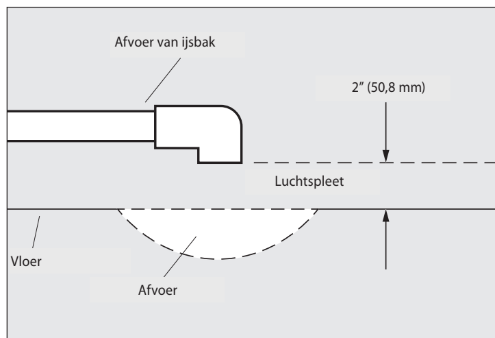
Afb. 2. Monteer afvoerleidingen altijd met een verticale luchtspleet van 50,8 mm (2 inch) tussen de vloer en het uiteinde van de leiding. De figuur is niet op schaal.
