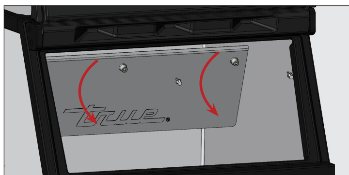
Afb. 2. Schuif de keerplaat naar achteren om deze te verwijderen.
