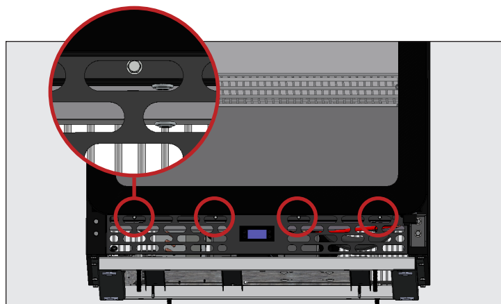
Afb. 3. Verwijder de voorste roosterbouten om toegang te krijgen tot de transportbouten.
