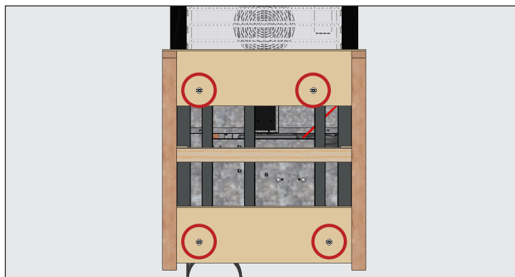
Afb. 2. Voorbeeld van de locaties van de transportbouten.
