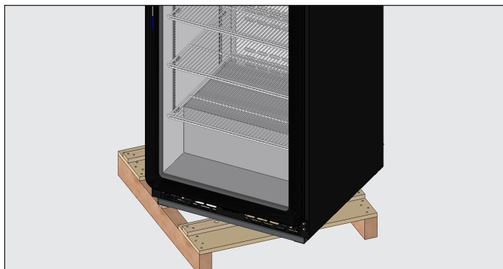
Afb. 4. Draai het apparaat op het pallet. Til de kast niet op aan het werkblad, de deuren, de laden of de roosters.
