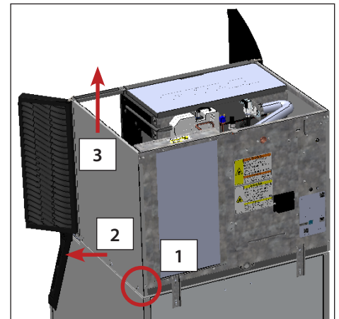
Рис. 3. Вывернуть винт, снять панель с язычков крепления, затем поднять и снять.
