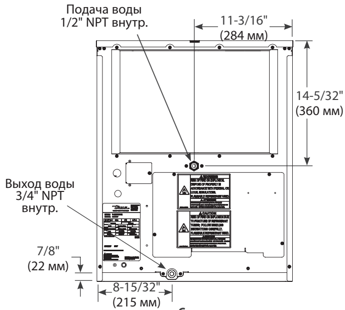
Сзади
