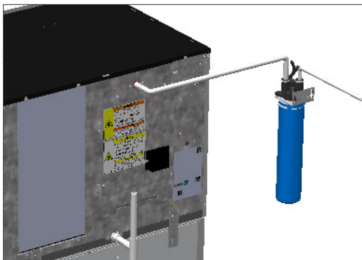
Рис. 1. Пример подключения к водопроводу сверху. Условия применения вашего устройства могут отличаться.
