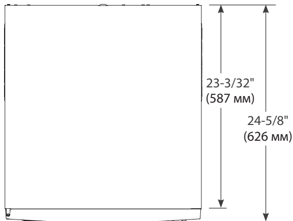
Сверху
