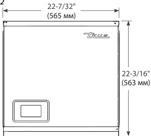
Спереди
