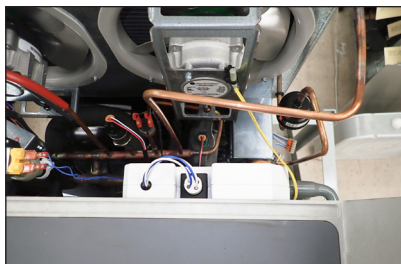
Рис. 2. УФ-система TRUEZONE, вид сверху.
