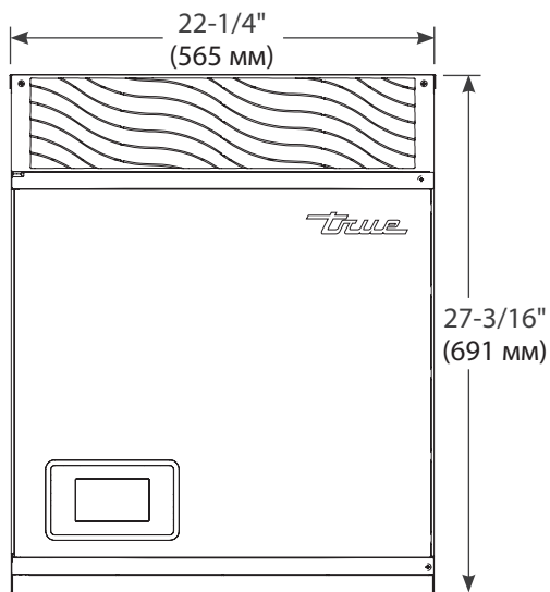
Спереди
