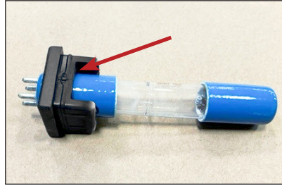
Fig. 4 Tacca della guarnizione di gomma.
