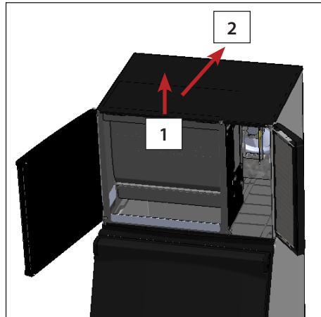
Fig. 2. Sollevare il bordo frontale, far scorrere indietro il pannello frontale, quindi sollevarlo per toglierlo.
