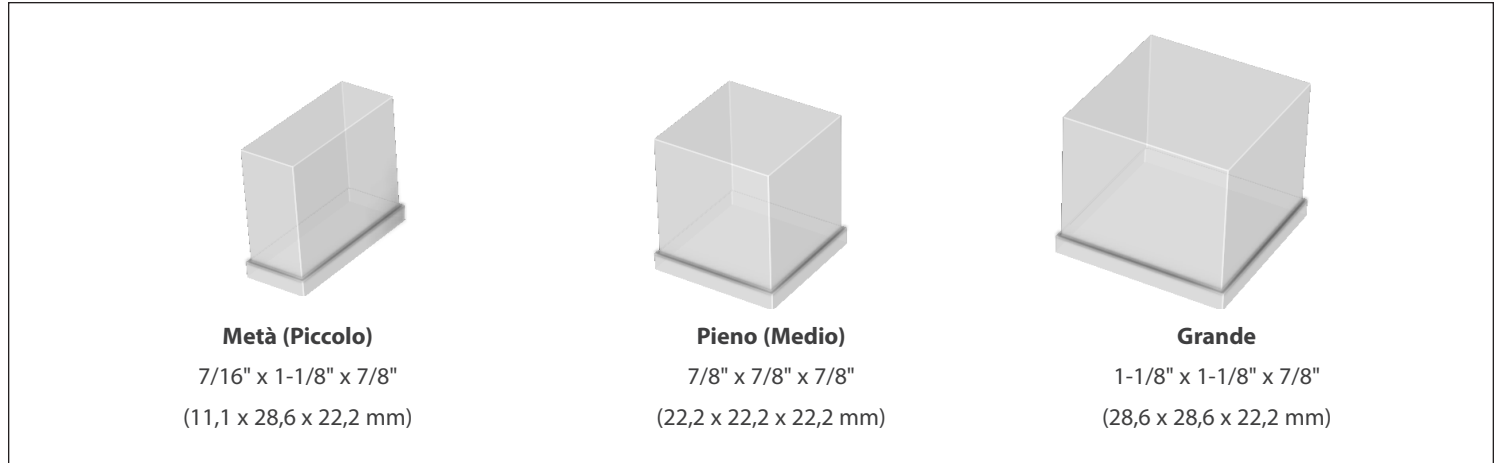
Fig. 1 Misure del cubetto e loro dimensioni.
