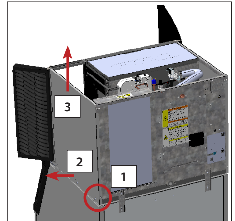
Fig. 3 Togliere le viti, tirare via il pannello dalle linguette aderenti, quindi sollevarlo per toglierlo.
