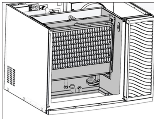
Vista frontale
