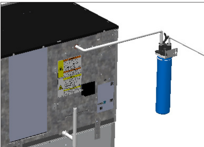
Fig. 1 Esempio di collegamento idraulico superiore. Il vostro elettrodomestico potrebbe essere diverso.
