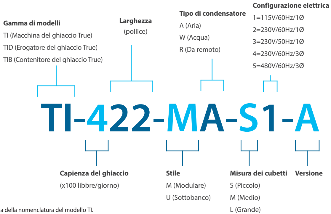
Fig. 1 Diagramma della nomenclatura del modello TI.
