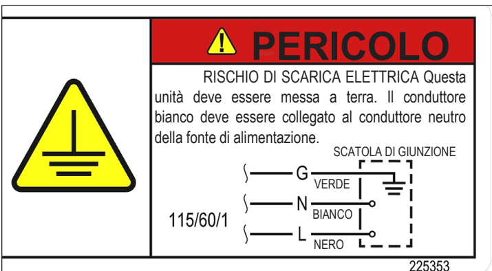
Fig. 4 Etichetta elettrica della scatola di giunzione.
