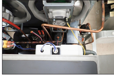
Abb. 2. Draufsicht des TRUEZONE UV-Systems.
