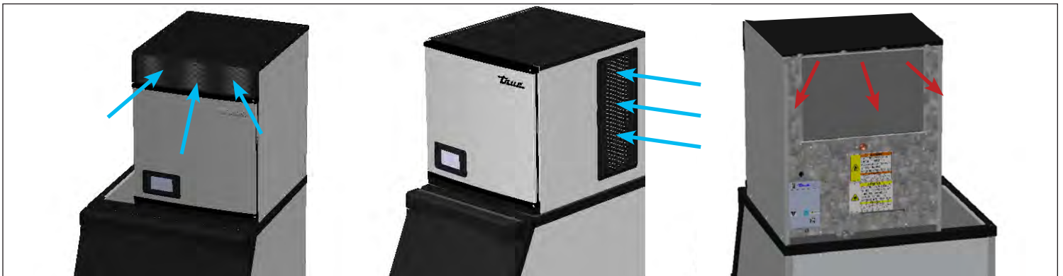
Fig. 2. El aire fluye hacia el frente y los costados, y sale por la parte trasera.
