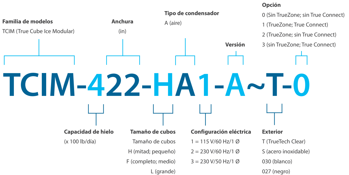
Fig. 2. Diagrama de nomenclatura del modelo TCIM.
