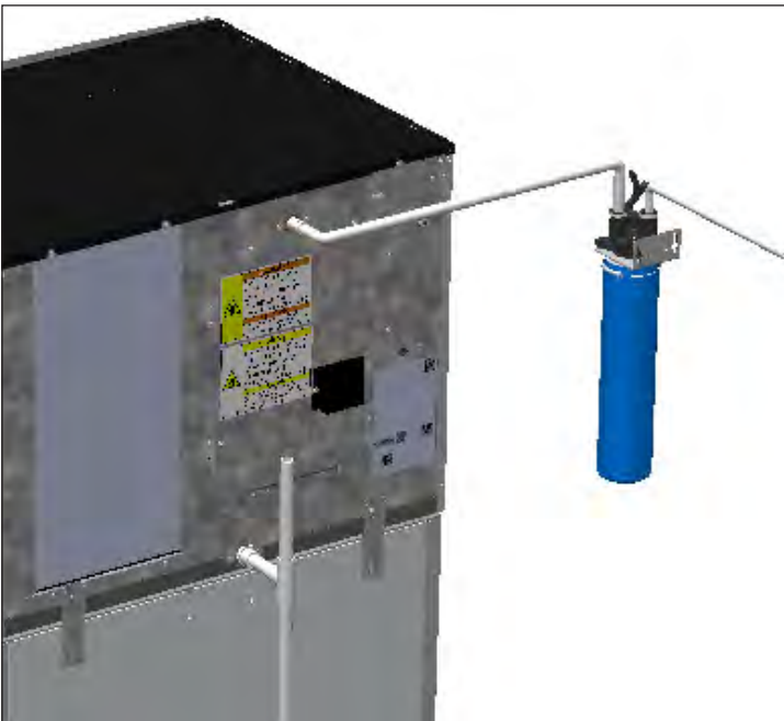
Fig. 1. Ejemplo de conexión de plomería en la parte superior. Su aplicación quizás sea distinta.
