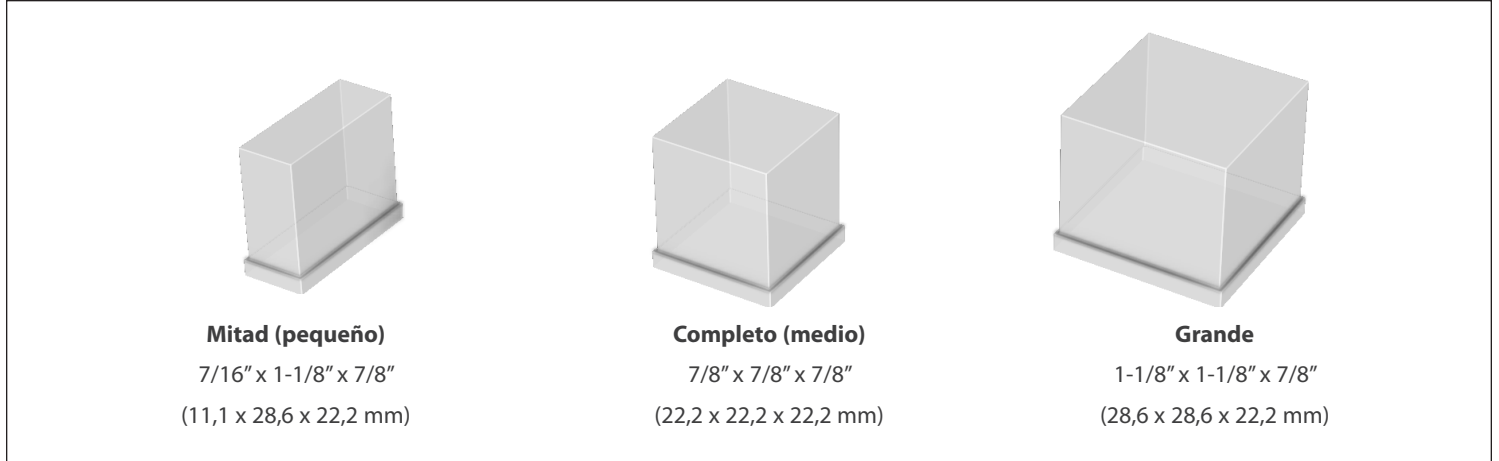
Fig. 1. Tamaños de cubos y sus dimensiones.
