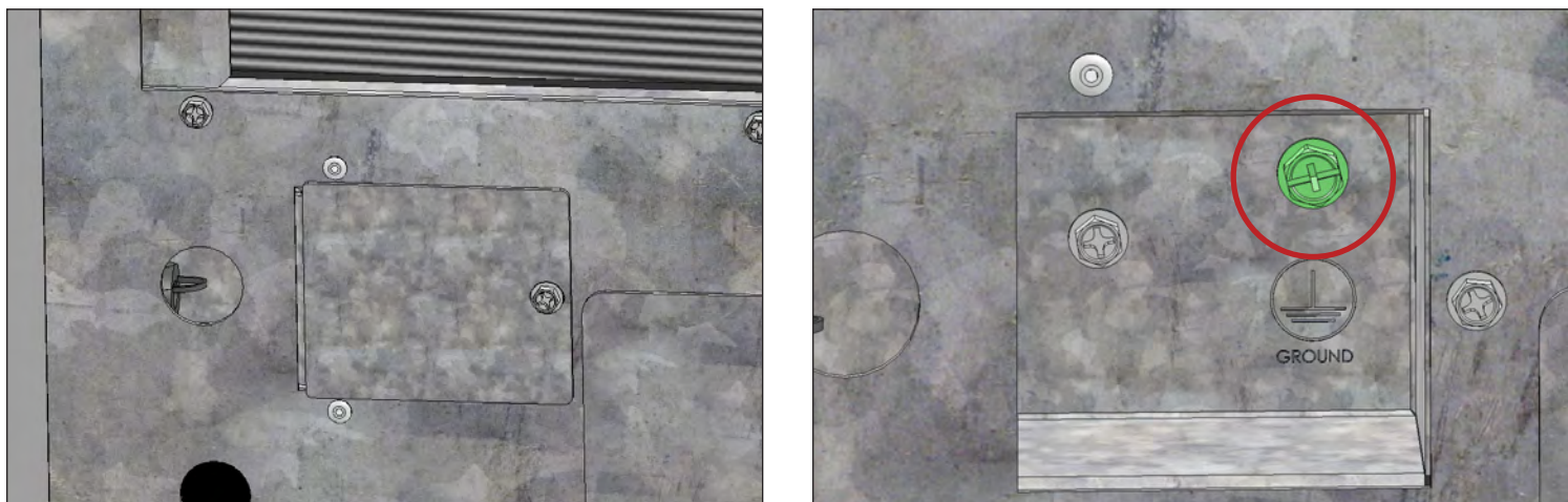
Рис. 3. Выполнить электрические соединения внутри соединительной коробки льдогенератора. Обязательно использовать устройства для снятия механического напряжения. Обязательно использовать зеленый винт заземления при выполнении электрических соединений.
