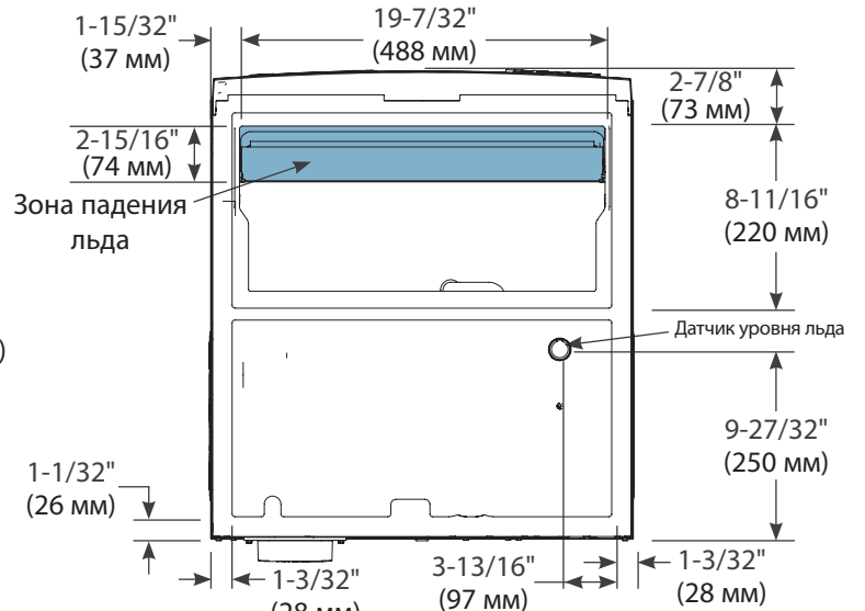
Снизу
