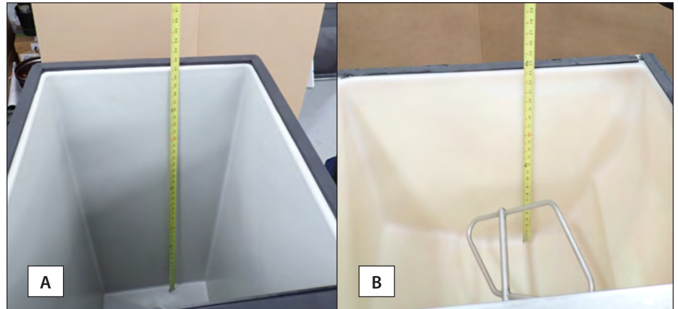
Рис. 2. Перед установкой льдогенератора обязательно измерить глубину контейнера (А) или диспенсера (В) для настройки датчика уровня льда.
