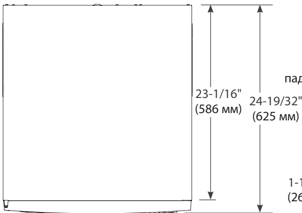
Сверху
