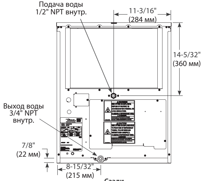
Сзади
