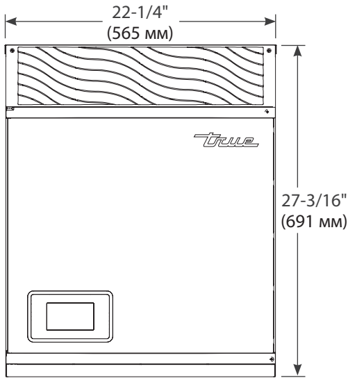
Спереди
