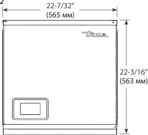
Спереди
