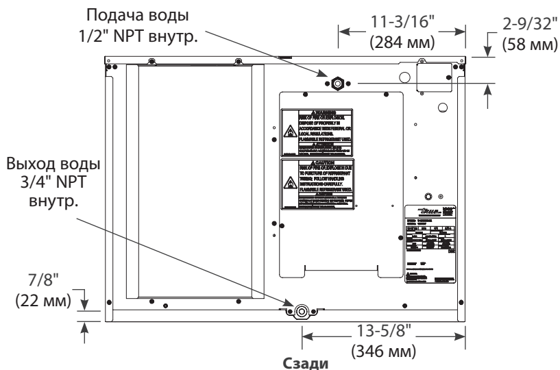
Сзади
