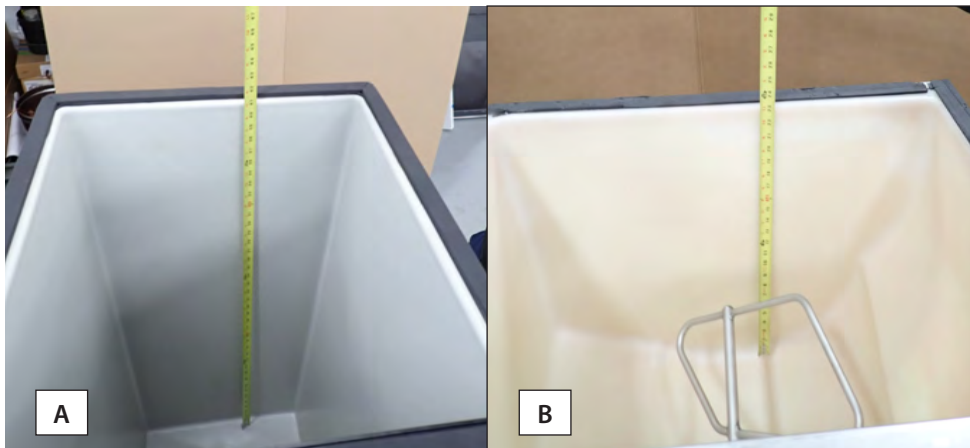
Rys. 2. Zawsze przed instalacją kostkarki do lodu wykonać pomiary zasobnika (A) lub dystrybutora (B) na potrzeby czujnika poziomu kostek lodu.
