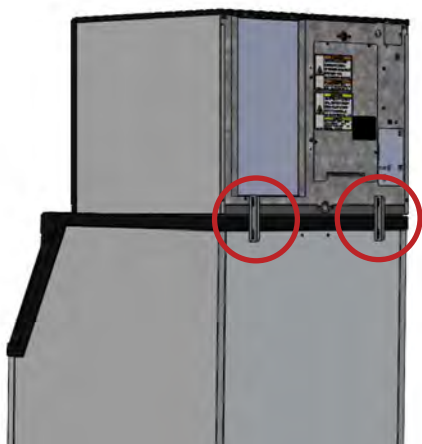
Rys. 1. Zamontować wsporniki zasobnika.
