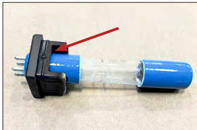
Rys. 4. Wgłębienie na gumowej uszczelce.
