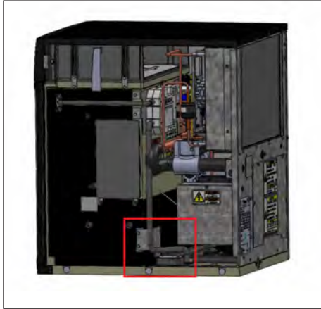
Afb. 1. Locatie van de ijsniveausensor.
