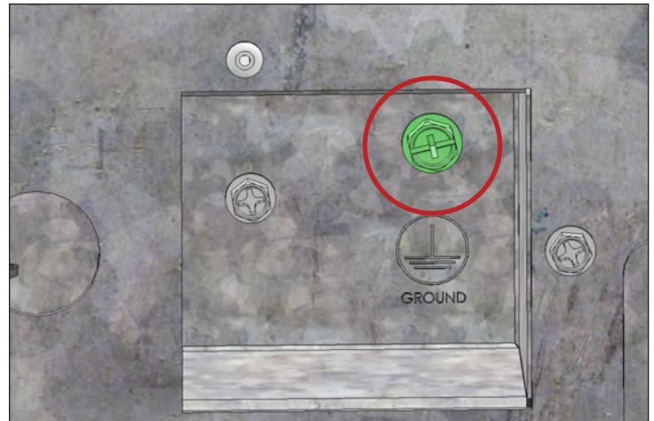
Afb. 3. Breng de elektrische aansluitingen aan in de verdeelkast van de ijsmachine. Zorg ervoor dat u trekontlastingen gebruikt. Gebruik altijd de groene aardingsschroef bij het maken van elektrische aansluitingen.
