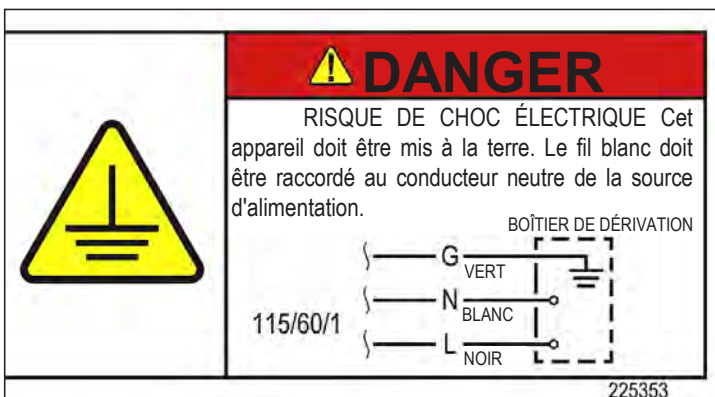
Fig. 4. Étiquette électrique de la boîte de dérivation.
