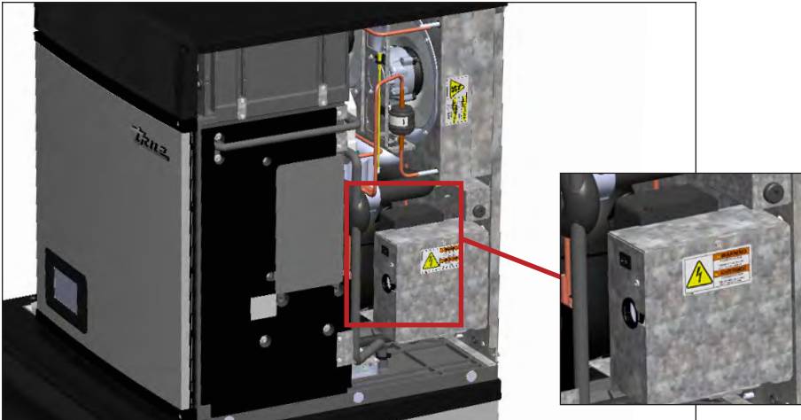
Fig. 2. Emplacement de l'interrupteur à bascule. L'interrupteur à bascule coupe l'alimentation de la carte de commande et de l'écran avant ; il ne coupe PAS l'alimentation de la totalité de l'appareil.
