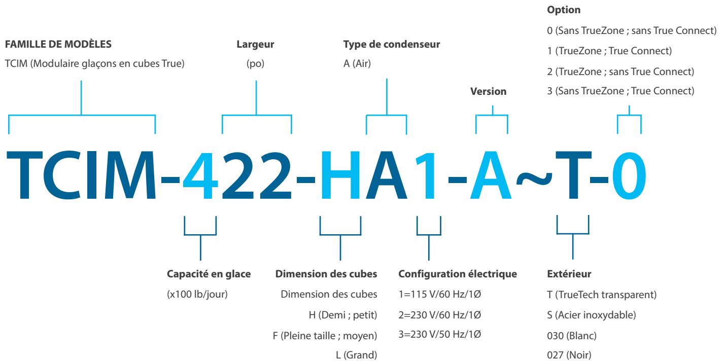
Fig. 2. Schéma de nomenclature du modèle TCIM.
