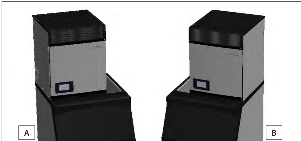
Fig. 3. Une machine à glaçons de 22" (560 mm) montée à gauche (A) et à droite (B) sur un bac de 30" (760 mm) avec un adaptateur de bac.
