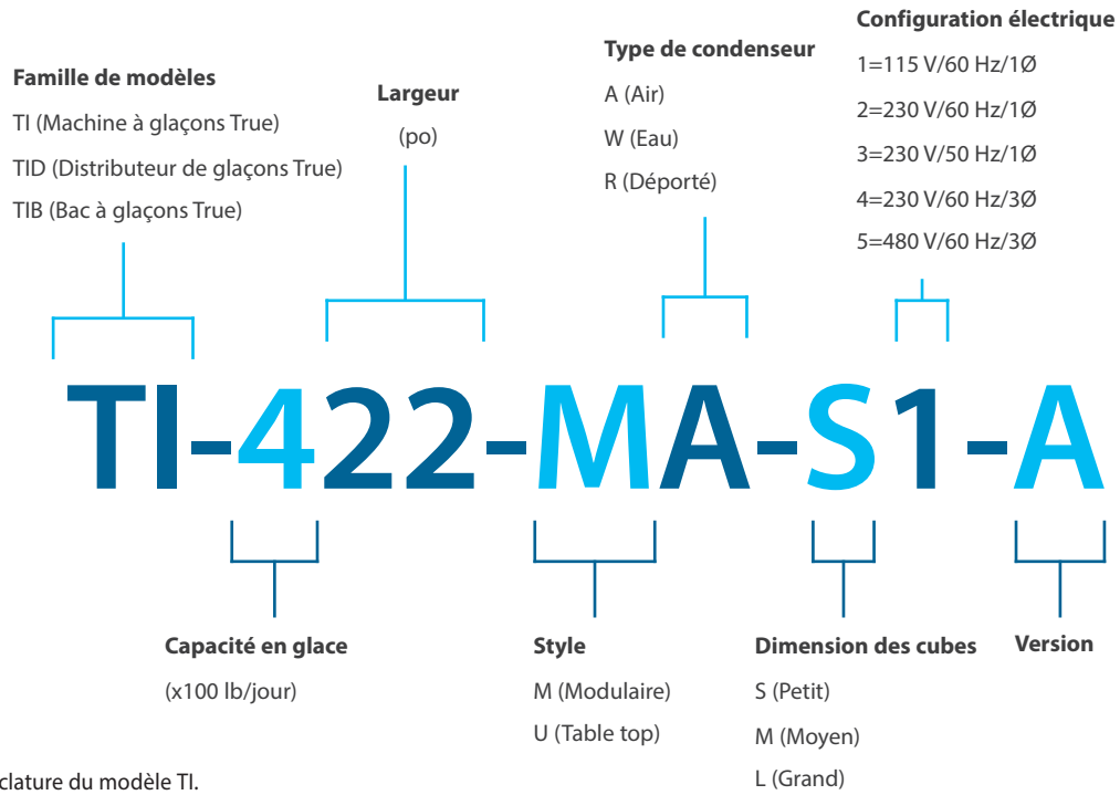
Fig. 1. Schéma de nomenclature du modèle TI.
