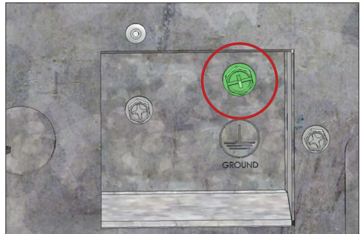
Fig. 3. Effectuez les raccordements électriques dans la boîte de dérivation de la machine à glaçons. Assurez-vous d'utiliser des presse-étoupes. Utilisez toujours la vis de terre verte pour les raccordements électriques.
