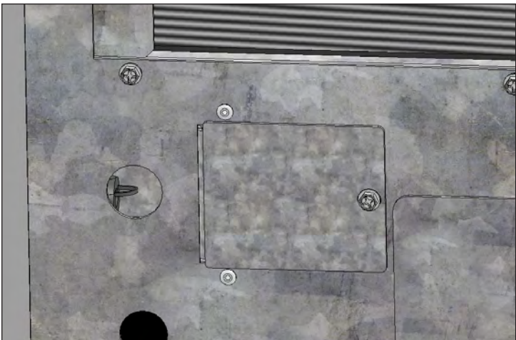
Fig. 3. Effectuez les raccordements électriques dans la boîte de dérivation de la machine à glaçons. Assurez-vous d'utiliser des presse-étoupes. Utilisez toujours la vis de terre verte pour les raccordements électriques.
