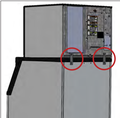
Fig. 1. Supports de bac installés.
