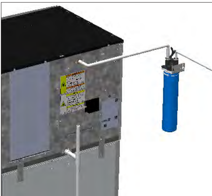
Fig. 1. Exemple de raccordements de plomberie par le haut. Votre application peut être différente.
