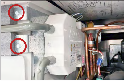
Fig. 3. Vue latérale du système UV TRUEZONE. Emplacements des vis du support TRUEZONE.
