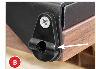
Fig. 5. Retirez la goupille et la douille de la charnière supérieure (A) et le support de la came de la porte (B) des supports de charnière. Ne retirez pas les supports de charnière.
