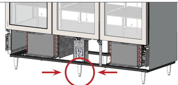
Rys. 2 Aby obniżyć urządzenie, nóżki poziomujące należy obracać w kierunku ruchu wskazówek zegara.
