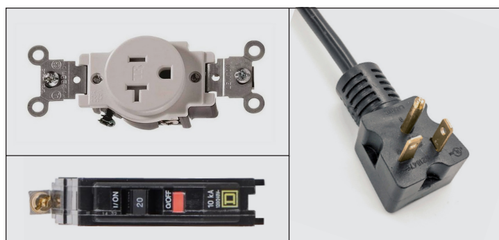
Rys. 2 Konfiguracja 3-przewodowa i wtyk czterobolcowy NEMA 5-20P/20R.
