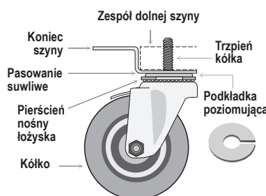
Rys. 7 Rozmieszczenie kółek.
